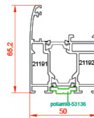
پروفیل لنگه Sash profiles
