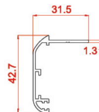
پروفیل روکوب ۴۲ Suppressed the bilding 10464 0.361 kg/m
