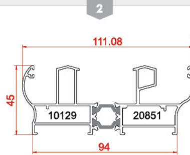
پروفیل فریم Frame profile 10129-20851 1.911 kg/m
