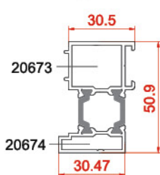
پروفیل آداپتور Adaptor profiles 20673-20674 1.047 kg/m
