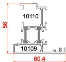
پروفیل وسط دولنگه The middle vent profiles 10109-10110 1.3 kg/m
