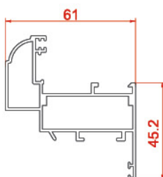
پروفیل لنگه کتیبه Vent for engraving profile 2609 1.10 kg/m
