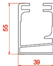
پروفیل ریل Rail Profiles 2887 1.420 kg/m
