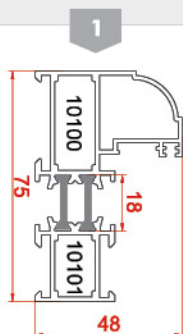
پروفیل فریم Frame profiles 10100-10101 1.6186 kg/m
