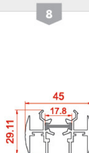
پروفیل وسط چهار لنگه profiles vent four middle The 20669-20669 0.911 kg/m
