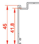
پروفیل روکوب Suppressed the bilding 20564 0.328 kg/m
