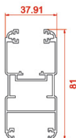
پروفیل لنگه طرحدار designs different with Vent 2602 1.2518 kg/m
