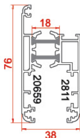
پروفیل لنگه زهواردار Vent with rickety 2811-20659 1.462 kg/m
