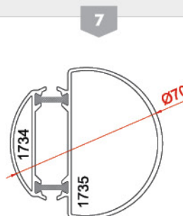
لوله محوری ترمال Axial tube thermal 1734-1735 1.544 kg/m
