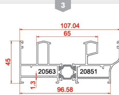
پروفیل فریم Frame profile 20563-20851 1.914 kg/m
