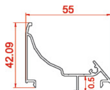
پروفیل گردان فریم profiles frame Rotating 10125 0.5459 kg/m
