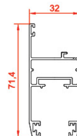
لنگه زهواردار Vent profile 21403 0.888 kg/m
