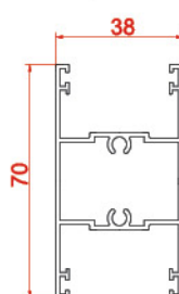
سپری بدون زهوار Tropetalous with out rickity Profil 21047 1.01 kg/m
