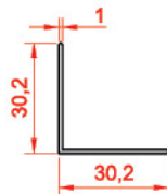
نبشی 30X30 20878 0.147
