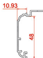
پروفیل روکوب Suppressed the binding 10319 0.421 kg/m
