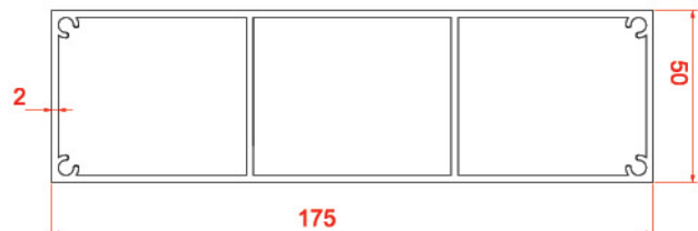
پروفیل لوور مستطیلی Rectangle Louvre
