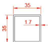
21653 0.649 kg/m
