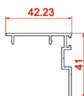
درپوش لنگه Caps for vent 21050 0.442 kg/m
