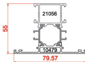
پروفیل سه پری فریم Tripetalous Profiles 10479-21056 1.183 kg/m
