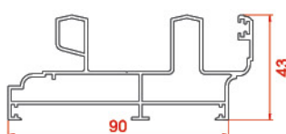
پروفیل فریم profiles Frame 2601 1.4818 kg/m
