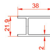
21648 0.542 kg/m
