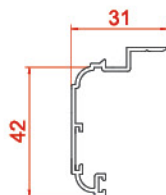
پروفیل روکوب ۴۲ Suppressed the binding 10467 0.391 kg/m
