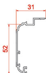
پروفیل روکوب ۵۲ Suppressed the bilding
