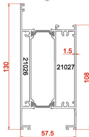
پروفیل پائین درب Low profile door 21026-21027 2.608 kg/m
