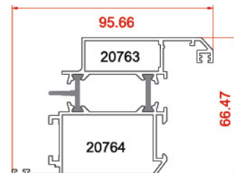
پروفیل لنگه جدید New Vent profiles 20763-20764 1.90 kg/m
