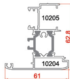
پروفیل وسط دولنگه profiles vent middle The 10204-10205 1.461 kg/m
