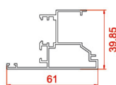
پروفیل وسط دولنگه The middle vent profiles 10137 0.7398 kg/m
