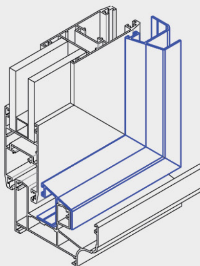
آبچکان کشویی AS 60
