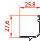
ریل توری Grid rails 20777 0.230 kg/m
