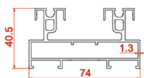
پروفیل فریم Frame profile 21048 1.368 kg/m
