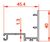
اینترلاک مونوریل Interlock
