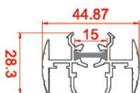
پروفیل وسط چهار لنگه The middle four door profiles 20699-20699 0.869 kg/m
