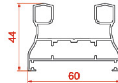
پروفیل فریم جدید profile frame new The 20657 0.990 kg/m
