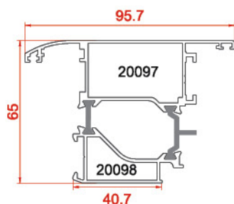
پروفیل لنگه بیرون بازشو درب vent opening side Out 20097-20098 1.855 kg/m
