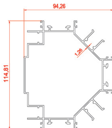
پروفیل پایه نود درجه سه طرفه By 90 Degrees Tripartite 20918 2.154 kg/m
