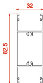
پروفیل سه پری Tripetalous profiles 2740 0.9423 kg/m
