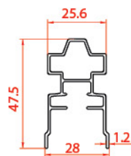
پروفیل لنگه باز شو Vent profile 21618 0.483 kg/m
