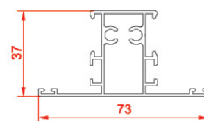
پروفیل سپری T profile 10411 0.7971 kg/m
