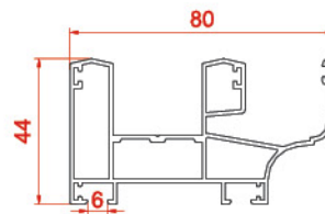
فریم پایین لاستیک خور frame on rubber a Place 20043 1.2985 kg/m
