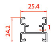
پروفیل ارتفاع فریم Frame height profile 21619 0.319 kg/m
