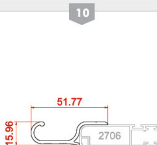
دستگیره لنگه توری Grid handle 21014 0.445 kg/m
