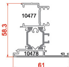
پروفیل وسط دو لنگه The middle vent 10477-10478 1.251 kg/m
