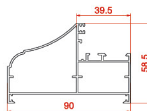
پروفیل کتیبه profiles Engraving 20062 1.2582 kg/m
