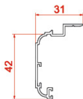
پروفیل روکوب ۴۲ Suppressed the bilding 10467 0.391 kg/m
