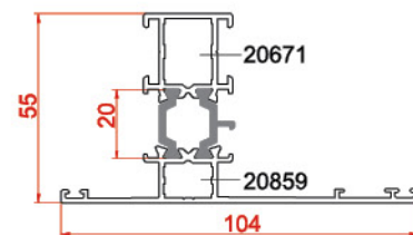
پروفیل سه پری Tripetalous profiles 20671-20859 1.411 kg/m
