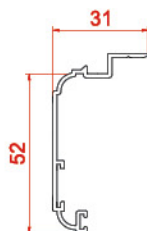
پروفیل روکوب ۵۲ Suppressed the blding 10466 0.428 kg/m
