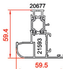
لنگه ی کرو Curved vent 20677-21593 1.339 kg/m
