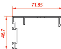
درپوش لنگه Gap for vent 20794 0.701 kg/m
