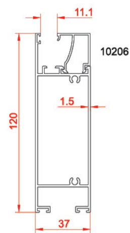
پروفیل پایین درب Low Profile Door 752 1.50 kg/m
