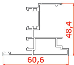
پروفیل وسط دولنگه Between Two Vent 783 0.880 kg/m
