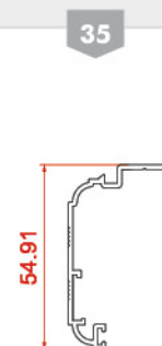
پروفیل روکوب Suppressed the binding 10319 0.422 kg/m
