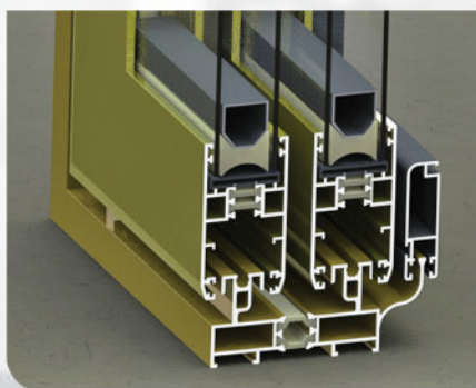
دیتیل لیست یراق آلات پنجره ترمال بریک کشویی TS 77 Thermal break sliding window fitting of series TS 77 (detail)
