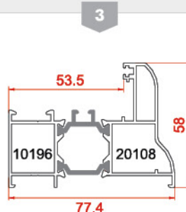
پروفیل کتیبه profiles Engraving 10196-20108 1.3992 kg/m
