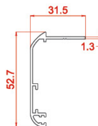
پروفیل روکوب ۵۲ Suppressed the bilding 10465 0.398 kg/m
