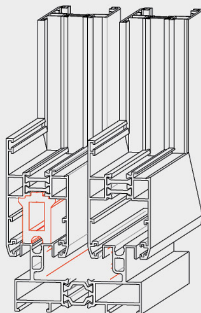
بالانسر پلاستیکی TS77 Code: 53023
