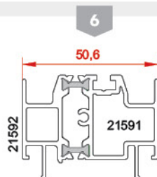
پروفیل وسط چهار لنگه Sliding sash adjoining profile 21591-21592 weight: 1.251 kg/m
