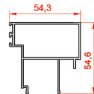
درپوش لنگه مخفی مونوریل Hidden vent cover
