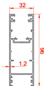
پروفیل لنگه Vent profile 21490 1.217 kg/m
