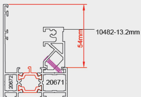
دیتیل نصب لقمه‌ی سپری 10482
