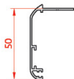
پروفیل روکوب Suppressed the binding 10465 0.391 kg/m
