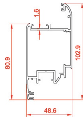
لنگه یراق یو پی وی سی ضخامت ۱.۶ Vent 1.6 10845 1.524 kg/m
