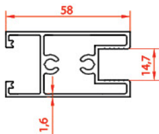
پروفیل ۶ سانتی 6cm profile 10811 1.168 kg/m
