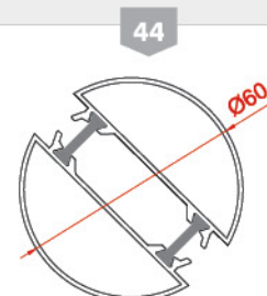
لوله محوری ترمال فریم ساده thermal tube Axial 20024-20024 1.787 kg/m
