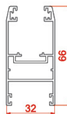
پروفیل لنگه profiles Vent 2741 0.9296 kg/m
