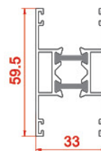
پروفیل سپری بدون زهوار Tripetalous without rickety 2798-2798 1.09 kg/m
