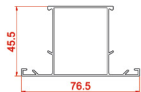
پروفیل سه پری Tripetalous profiles 182 0.690 kg/m
