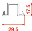
زهوار تک جداره Rickety for Single-walled glass 735 0.2957 kg/m
