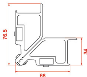
فیکسر زیر دکمه پلاستیک
