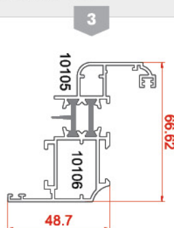
پروفیل لنگه Vent profiles 10105-10106 1.4734 kg/m
