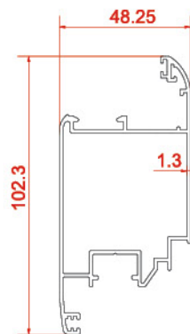
پروفیل یراق یو پی وی سی لنگه درب Door vent profiles 20860 1.263 kg/m
