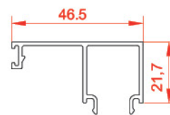
درپوش فریم مونو ریل caps for frame 21625 weight: 0.432 kg/m
