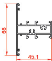
پروفیل سپر T profile
