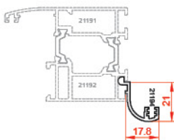
پروفیل آببندی Cap water-proofing
