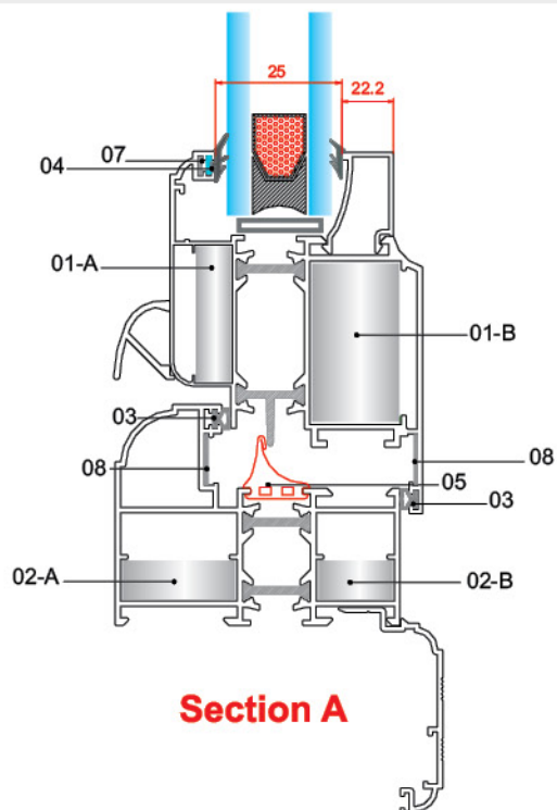
دیتیل یراق آلات درب لولایی ترمال بریک سری TH 75H Thermal break hinged door fittings of series TH 75H (detail)
