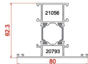
پروفیل سه پری لنگه Tripetalous Profiles 20793-21056 1.438 kg/m
