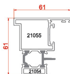
پروفیل آداپتور محوری Pivot adaptor profiles 21055-21054 1.549 kg/m
