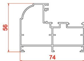
پروفیل کتیبه Engraving profile 2607 1.253 kg/m
