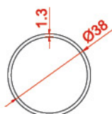
لوله محوری ۳۸ The central tube 38 20746 0.426 kg/m
