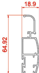
لنگه توری Grid Vent 21076 0.634 kg/m
