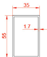
21652 0.842 kg/m
