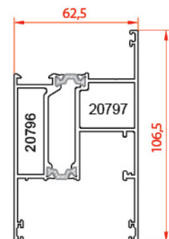
لنگه مونو ریل Vent profiles 20796-20797 2.216 kg/m
