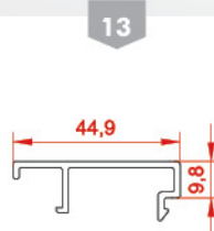
درپوش سه لنگه وسط باز شو cap for three sash sliding 21642 0.373 kg/m
