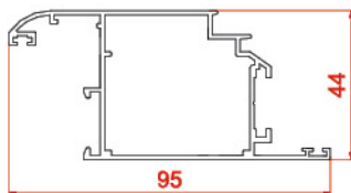
پروفیل لنگه درب Vent for door 20745 1.1 kg/m
