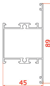
پروفیل سپری Tripetalous Profiles 749 1.08 kg/m
