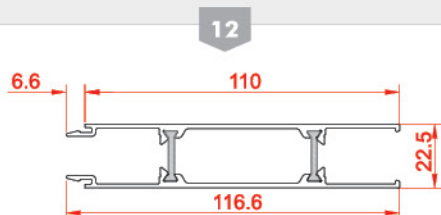
ورق دوجداره‌ی ترمال بریک Thermal break facade 21832-21832 1.422 kg/m
