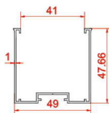
کاور قوطی آهنی ۴۰ × ۸۰ Gap for Iron Box 40x80 20778 0.490 kg/m
