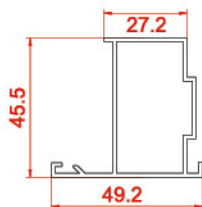
پروفیل باز شو محوری Axial opening profiles 267 0.6762 kg/m
