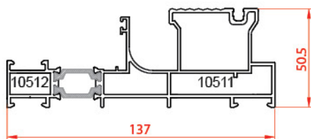
فریم مونو ریل Sliding - fix frame 10511-10512 2.525 kg/m
