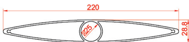
پروفیل لوور بیضی oval louvre code: 21535 weight: 2.851 kg/m
