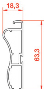
لنگه توری grid vent 21533 weight: 0.29 kg/m
