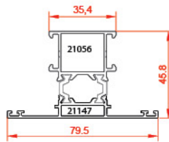
پروفیل T T profiles
