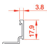
زهوار فریم مونو ریل glazing bid on fix 21623 weight: 0.179 kg/m
