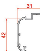
پروفیل روکوب ۴۲ Suppressed the bilding 10467 0.391 kg/m
