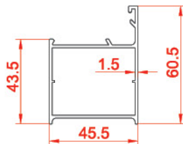
پروفیل فریم Frame profile 20194 0.885 kg/m
