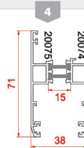
پروفیل لنگه profiles Vent 20075-20074 1.055 kg/m
