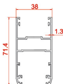
لنگه بدون زهوار Vent with out rickity 21051 1.011 kg/m
