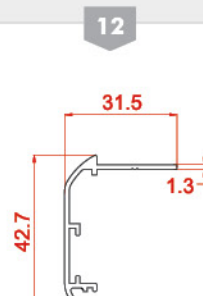
پروفیل روکوب ۴۴ Suppressed the bilding 10464 0.361 kg/m
