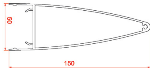
پروفیل ابتدا و انتهای لوور Profiles at the begining and end
