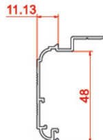
روکوب صاف Suppressed the binding 10248 0.4165 kg/m
