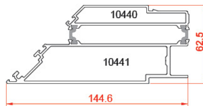
پروفیل زاویه 90 Corners profiles 10440-10441 3.301 kg/m
