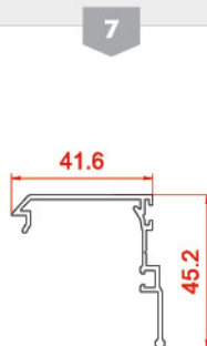
درپوش Gap 20067 0.4346 kg/m
