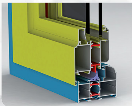
دیتیل یراق آلات درب لولایی ترمال بریک سری TH 75H Thermal break hinged door fittings of series TH 75H (detail)
