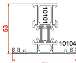
پروفیل سپری Tripetalous profiles 10104-10101 1.3674 kg/m
