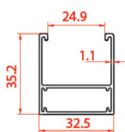
پروفیل عرض فریم Frame width profile 21616 0.455 kg/m
