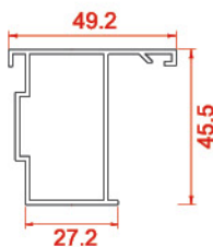
پروفیل باز شومحوری Axiyal opening profiles 267 0.6762 kg/m
