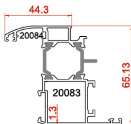
لنگه پنجره Vent rofiles 20084-20083 1.501 kg/m
