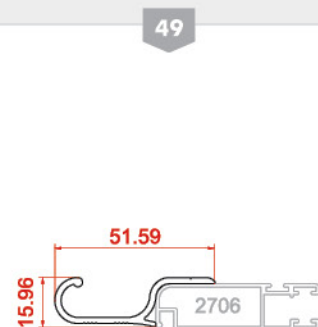
دستگیره لنگه توری Grid handle 21014 0.445 kg/m
