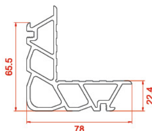
فیکسر پانچی
