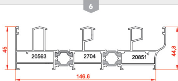
پروفیل فریم سه ریل 3 Rail frame 20563-2704-20851 2.66 kg/m
