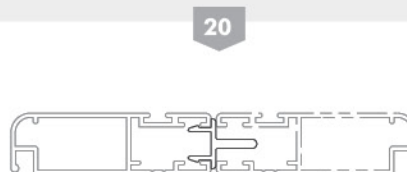
مابین چهار لنگه ی توری ریلی Sliding adjoining profile for fly-screen sash 10516 0.149 kg/m
