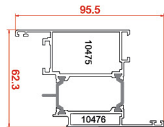
لنگه درب Door vent 10475-10476 1.631 kg/m
