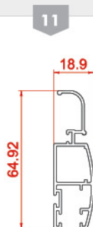
لنگه توری vent Grid 21076 0.634 kg/m
