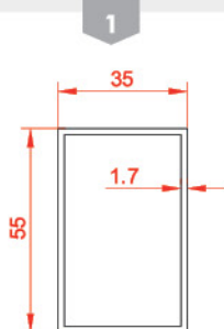
قوطی ۳۵ x ۵۵ Box 35x55 21652 0.842 Kg/m
