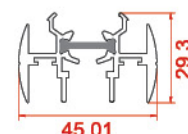
وسط چهار لنگه The middle four vent profile 20669-20669 0.869 kg/m
