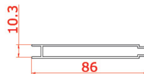
ورق دو جداره Double Sheet 115 0.6455 kg/m
