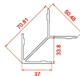
فیکسر آلدوکس سنگین
