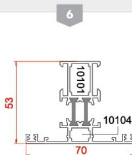
پروفیل سه پری Tripetalous profiles 10104-10101 1.3674 kg/m
