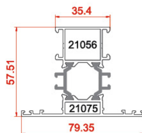
پروفیل سه پری و فریم محوری Pivot frame profiles 21056-21075 1.451 kg/m
