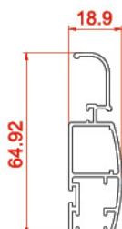
لنگه توری Grid Vent
