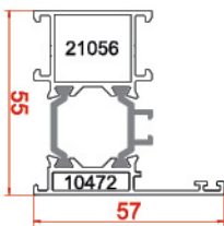
پروفیل فریم Frame Profiles 10472-21056 1.221 kg/m
