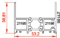
پروفیل کتیبه Cornice profiles
