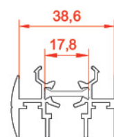
وسطی چهار لنگه Sliding sash adjoining profile 20669-20669 weight: 0.911 kg/m
