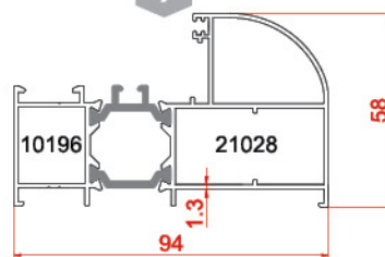
پروفیل کتیبه Engraving profile 10196-21028 1.773 kg/m
