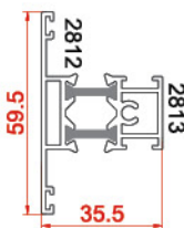
پروفیل سپری برای ۲۸۱۱-۲۸۱۲ Tripetalous with rickety 2813-2812 0.936 kg/m
