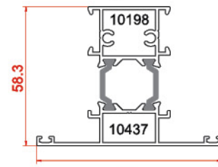
سپری درب بیرون باز شو Tripetalous profiles 10437-10198 1.48 kg/m
