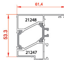
آداپتور بیرون بازشوی درب Outside opening adaptor 21247-21248 1.375 kg/m
