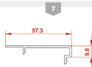
اینتر لاک interlock profile 21586 weight: 0.357 kg/m
