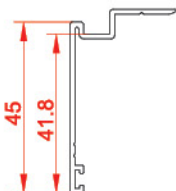
پروفیل روکوب Suppressed the blding 20564 0.328 kg/m
