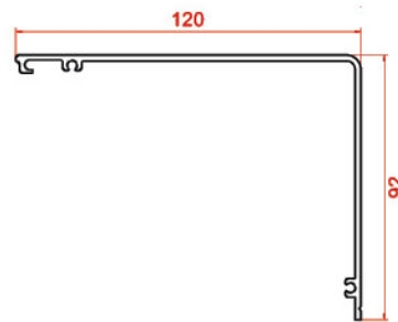
پروفیل کاور Rail profile 20781 1.287 kg/m
