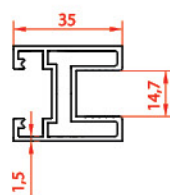
پروفیل ۳/۵ سانتی کناری 3.5cm profile 10812 0.778 kg/m
