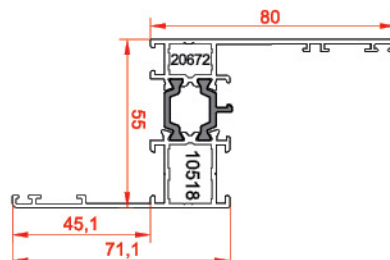
فریم روکوب دار Frame profile 20672-10518 1.589 kg/m
