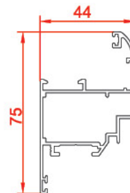
لنگه متوسط Vent profiles 21205 0.947 kg/m
