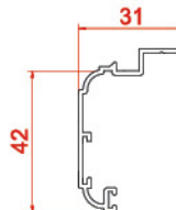
پروفیل روکوب ۴۲ Suppressed the blding 10467 0.391 kg/m
