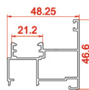
پروفیل وسط دو لنگه The middle vent 20844 kg/m 0.665
