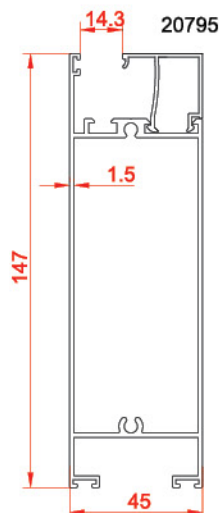
پروفیل پایین درب Low Profile Door 750 1.8444 kg/m
