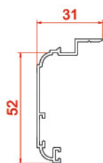
پروفیل روکوب ۵۲ Suppressed the bilding 10466 0.428 kg/m
