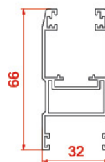
پروفیل لنگه طرحدار designs different with Vent 10116 0.9391 kg/m
