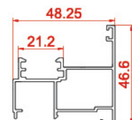
پروفیل وسط دو لنگه The middle vent 20844 0.665 kg/m
