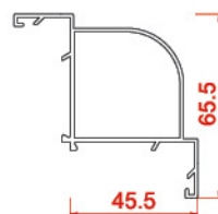
پروفیل گردان فریم Rotating frame profiles 165 0.8045 kg/m
