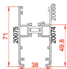
لنگه ی بازو کشویی vent profile 20074-20075 weight: 1.055 kg/m
