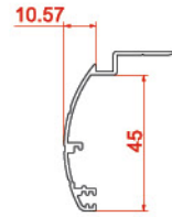
روکوب گرد Suppressed the binding 10117 0.380 kg/m
