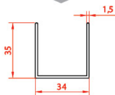
پروفیل یو شکل U profile 10815 0.431 kg/m
