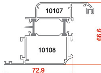
پروفیل لنگه Vent profiles 10107-10108 1.8952 kg/m
