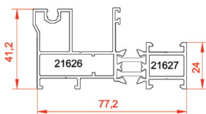
فریم مونو ریل frame mono rail 21626-21627 weight: 1.513 kg/m
