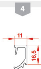
پروفیل زهوار رنگ پودری Glazing bead 21587 weight: 0.212 kg/m
