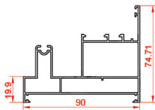
پروفیل مونوریل Monorail Profiles
