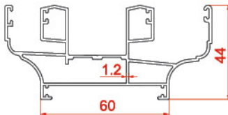
فریم دارای عرق گیر IfiFrame Pro 20853 1.503 kg/m
