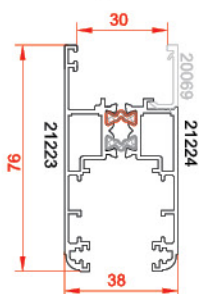
پروفیل لنگه زهواردار Vent with rickety 21223-21224 1.462 kg/m
