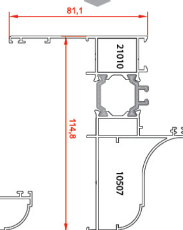
فریم روکوب دار Frame Profiles 10507-21010 2.011 kg/m
