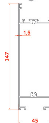
پروفیل پایین درب Low Profile Door 750 1.8444 kg/m
