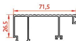
درپوش مونو ریل Slidin-fix cap 10513 0.819 kg/m
