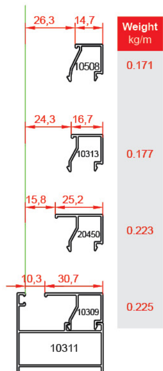
دیتیل یراق آلات پنجره آلدوکس سبک AH45L طرح ایران Lightweight window aldoks fitting of series AH 45L Iran plans (detail)
