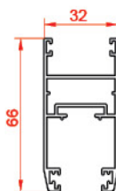
پروفیل لنگه Sash profiles
