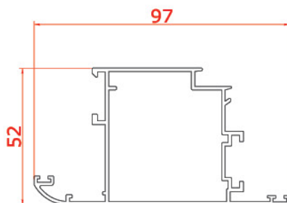
پروفیل لنگه بیرونی باز شو Outside Opening vent 10304 1.184 kg/m
