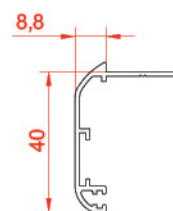
پروفیل رکوب ۴۲ Trimming profile 10464 weight: 0.361 kg/m
