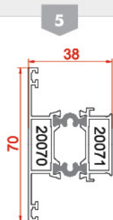
پروفیل سه پری Tripetalous profiles 20070-20071 1.007 kg/m
