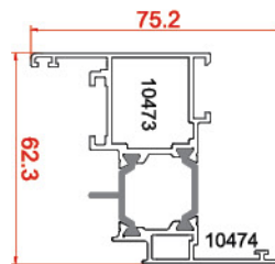
لنگه پنجره Vent Profiles 10473-10474 1.289 kg/m
