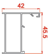
پروفیل فریم Frame profiles 180 0.4718 kg/m
