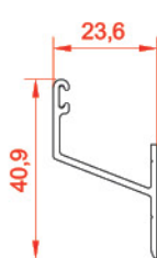
ریل توری مونو ریل rail profil 21629 weight: 0.285 kg/m
