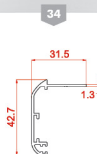
پروفیل روکوب ۴۲ Suppressed the binding 10464 0.361 kg/m
