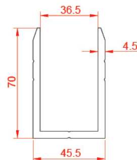
10435 2.211 kg/m
