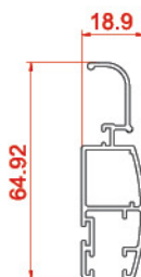
لنگه توری Grid vent 21076 0.634 kg/m
