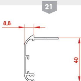
پروفیل رکوب Trimming profile 10464 weight: 0.361 kg/m
