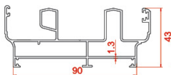
پروفیل فریم Iupro Frame 20852 1.712 kg/m
