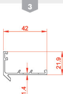
فریم نصب شیشه Fix Frame Profile 21654 0.357 Kg/m
