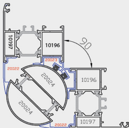
پروفیل لوله محوری 20024-20022 فقط در فریم 10196-10197 کاربرد دارد.
