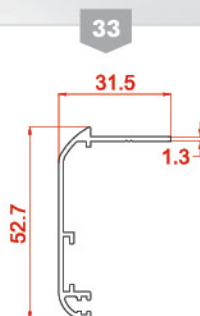
پروفیل روکوب ۵۲ Suppressed the binding 10465 0.398 kg/m
