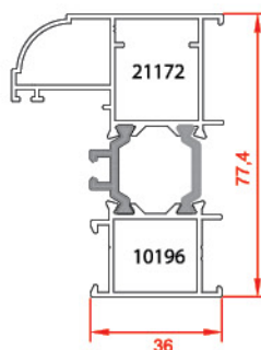
لنگه ی بادبزدی Vent Profiles 10196-21172 1.478 kg/m
