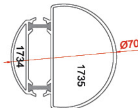
لوله محوری ترمال Axial tube thermal 1734-1735 1.544 kg/m
