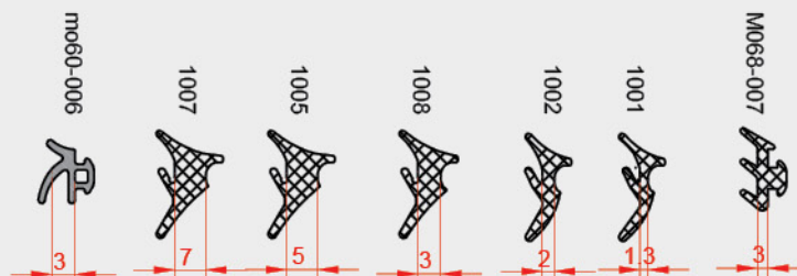
اندازه ی شیشه و لاستیک ها
