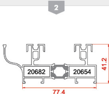
پروفیل فریم جدید profiles frame New 20682-20654 1.7494 kg/m
