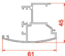
پروفیل وسط دولنگه The middle vent profiles 760 0.7674 kg/m
