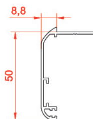
پروفیل رکوب ۵۲ Trimming profile 10465 weight: 0.398 kg/m
