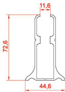
شیشه گیر Glass Holder 822 1.495 kg/m
