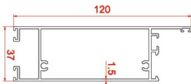
پروفیل پایین درب Low profile door 752 1.5 kg/m
