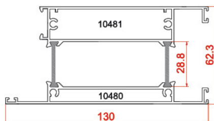
پروفیل پایین درب Low profile door 10480-10481 2.611 kg/m
