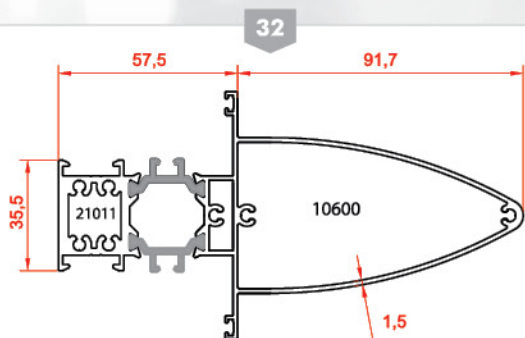
پروفیل سه‌پری تقویت شده Tripetalous profiles 21011-10600 2.849 kg/m
