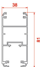
پروفیل لنگه profiles Vent 2742 1.1766 kg/m
