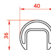
پروفیل شیشه گیر Glass hand rail
