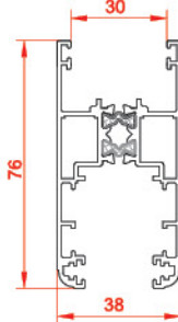
پروفیل لنگه ی جدید بدون زهوار New vent profiles 21223-21223 1.376 kg/m
