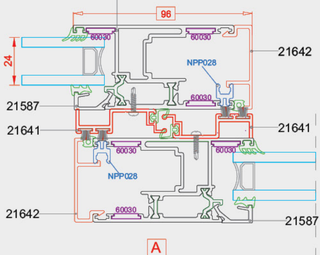
سه لنگه وسط باز شو Lift & Slide
