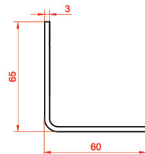
پراکت 65X60 21221 1.02
