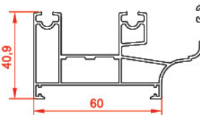
پروفیل فریم leftFrame Pro 10510 1.227 kg/m
