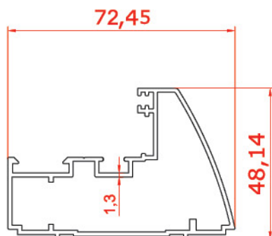
پروفیل فریم درب Frame Profiles 20921 1.008 kg/m
