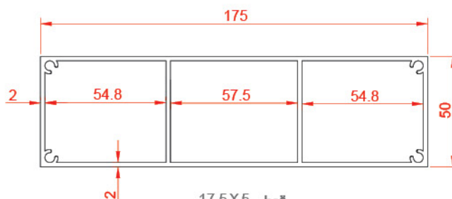
قووطى 17.5X5 21061 3.379 kg/m
