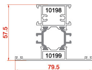
پروفیل سه پری Tripetalous profiles 10198-10199 1.499 kg/m
