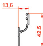
پایه توری لولایی Sliding fly-screen sash rail
