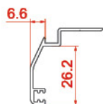
روکوب ۳ سانتی Suppressed the binding 20031 0.2724 kg/m
