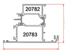
پروفیل بیرون باز شو درب Out side opening vent 20782-20783 1.82 kg/m
