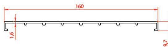
پروفیل کاور نما Cover profile 10817 0.921 kg/m
