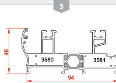
پروفیل فریم Frame profile 3580-3581 1.887 kg/m
