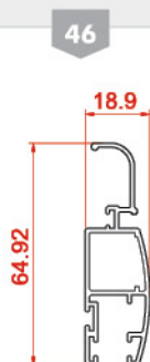
لنگه توری Grid vent 21076 0.634 kg/m
