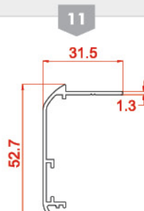
پروفیل روکوب ۵۲ Suppressed the bilding 10465 0.398 kg/m
