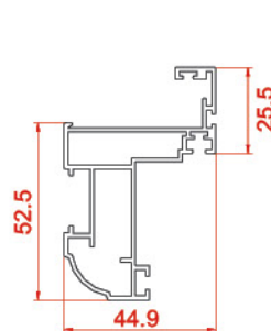
پروفیل یک جداره ثابت Fixed Single-walled profiles 10115 0.9847 kg/m
