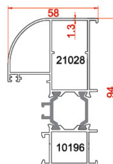
فریم بزرگ ۹۴ Frame Profiles 21028-10196 1.771 kg/m
