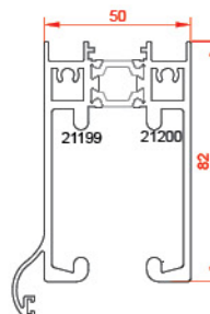
فریم بالا Cornice profiles
