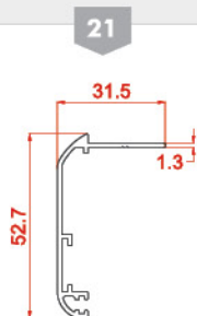
پروفیل روکوب ۵۲ Suppressed the blding 10465 0.398 kg/m
