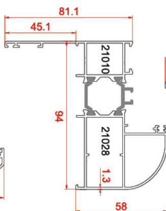
فریم روکوب دار Frame Profiles 21010-21028 1.951 kg/m
