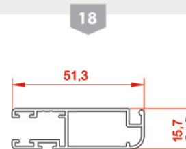
درپوش سه لنگه وسط باز شو cap for three sash sliding 21641 0.386 kg/m
