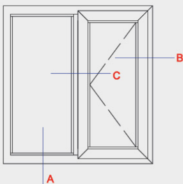
دیتیل یراق آلات پنجره آلدوکس سبک AH45L طرح ایران Lightweight window aldoks fitting of series AH 45L Iran plans (detail)
