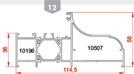
پروفیل کتیبه FRAME PROFILES 10196-10507 1.792 kg/m
