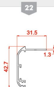
پروفیل روکوب ۴۲ Suppressed the blding 10464 0.361 kg/m
