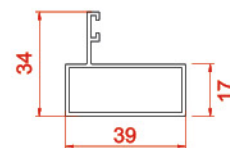
پروفیل کناری Lateral Profiles 2888 0.4568 kg/m
