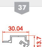
پروفیل گردان فریم profiles frame Rotating 20023 0.23 kg/m
