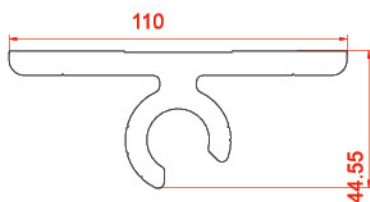
پروفیل پایه لوور Basic Louvre
