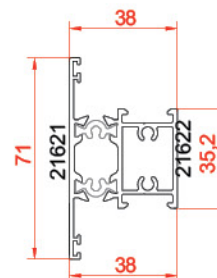
سپری برای فریم مونو ریل T profile 21621-21622 weight: 1.241 kg/m
