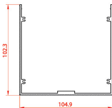
پروفیل یو شکل داخل سطح U Case profile
