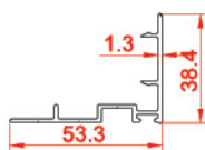
اینترلاک لنگه inter lock profile 21495 0.442 kg/m
