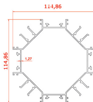
پروفیل پایه نود درجه چهار طرفه By 90 Degrees Bilaterally 20929 2.476 kg/m
