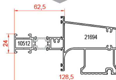
کتیبه ی مونوریل engraving profile 10512-21649 2.661 kg/m
