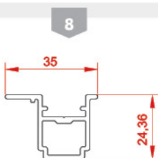
پروفیل نصب و تسمه دستگیره Accessory profile 21588 weight: 0.467 kg/m
