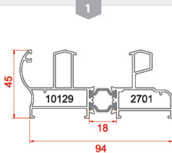
پروفیل فریم Frame profiles 10129-2701 1.725 kg/m
