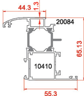
پروفیل لنگه متوسط profiles vent Average 10410-20084 1.50 kg/m
