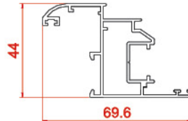
لنگه پراق یو پی وی سی خور پنجره Vent profiles with upvc fitting for window 20757 0.895 kg/m
