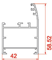
پروفیل فریم Frame profiles 20743 0.766 kg/m
