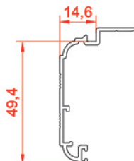
پروفیل رکوب Trimming profile 10318 weight: 0.399 kg/m
