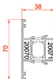
سپری برای لنگه کشویی T profile 20070-20071 weight: 1.007 kg/m
