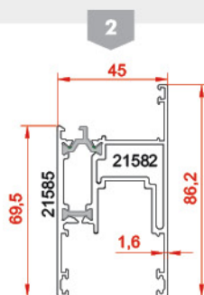
پروفیل لنگه vent profile 21582-21585 weight: 1.695 kg/m
