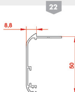
پروفیل رکوب Trimming profile 10465 weight: 0.391 kg/m
