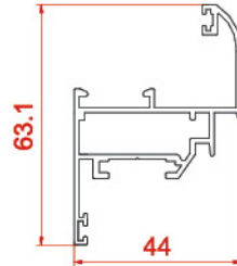
پروفیل لنگه Vent profiles 20744 0.802 kg/m
