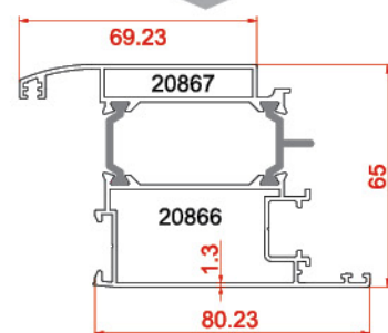
لنگه یراق پی وی سی درب Door vent 20867-20866 1.899 kg/m
