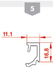
پروفیل زهوار انادایز Glazing bead 21640 weight: 0.268 kg/m
