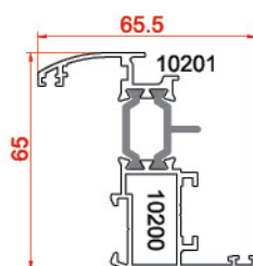
پروفیل لنگه کوچک profiles vent Small 10200-10201 1.254 kg/m
