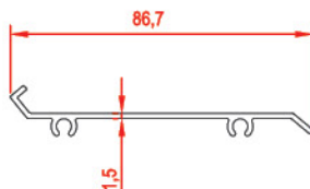
پروفیل منفذ Pore profile
