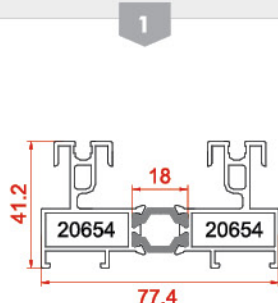
پروفیل فریم جدید profiles frame New 20654-20654 1.6061 kg/m
