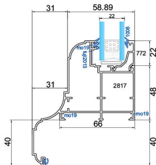
پروفیل ویتترین 59K
