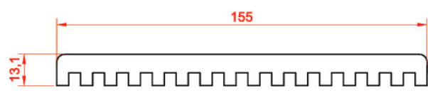
پروفیل 155X13 21246 4.641
