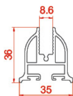
شیشه گیر پا فکی Glass Stack 2886 09116 kg/m
