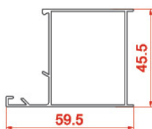
پروفیل فریم Frame profiles 183 0.5914 kg/m
