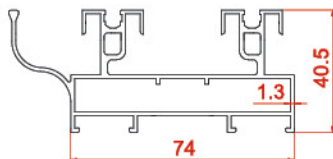
پروفیل فریم Frame profile 21052 1.522 kg/m
