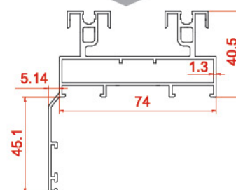
پروفیل فریم روکوبدار Frame profile 21057 1.597 kg/m
