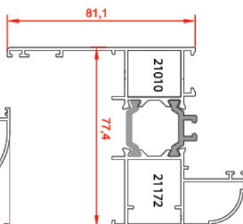
فریم روکوب دار Frame Profiles 21010-21172 1.692 kg/m
