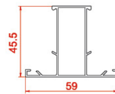
پروفیل سه‌پری Tripetalous profiles 179 0.5893 kg/m
