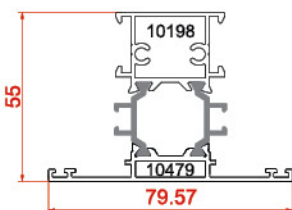
پروفیل سه پری فریم Tripetalous Profiles 10479-10198 1.467 kg/m
