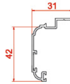
پروفیل روکوب ۴۲ Suppressed the bilding 10467 0.391 kg/m
