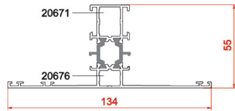
پروفیل سه پری Tripetalous profiles 20676-20671 1.84 kg/m
