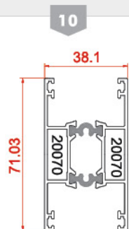
سه پری بدون زهوار rickety without Tripetalous 20070-20070 1.122 kg/m
