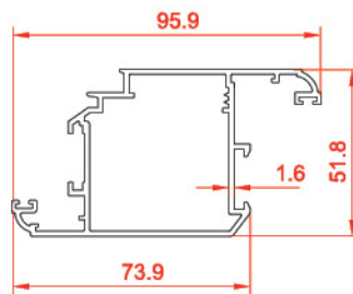
لنگه درب ضخامت ۱.۶ Frame profiles 10844 1.451 kg/m
