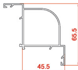
پروفیل گردان فریم Rotating frame profile 165 0.8045 kg/m
