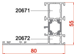
پروفیل فریم Frame profiles 20671-20672 1.44 kg/m
