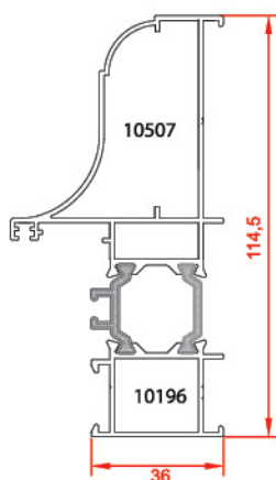
فریم Frame Profiles 10196-10507 1.792 kg/m
