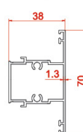
سپری زهواردار Tropetalous with rickity 21046 0.829 kg/m
