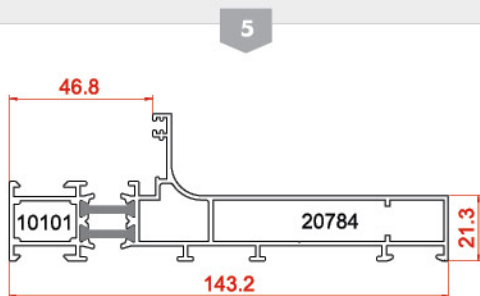
پروفیل فریم Frame Profiles 10101-20784 1.48 kg/m
