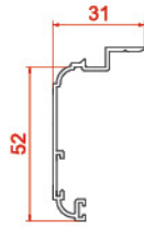
پروفیل روکوب ۵۲ Suppressed the bilding 10466 0.428 kg/m
