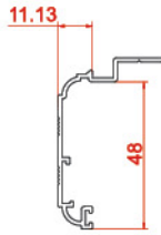
روکوب صاف Suppressed the binding 10248 0.4165 kg/m
