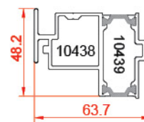
پروفیل وسط چهار لنگه the middle four vent 10438-10439 1.601 kg/m
