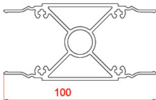
پروفیل لوور میانی Middle Louvre
