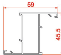
پروفیل لنگه Vent profiles 178 0.5893 kg/m
