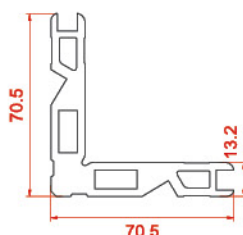
فیکسر پانچی
