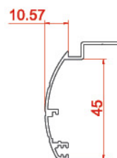
روکوب گرد Suppressed the binding 10117 0.380 kg/m
