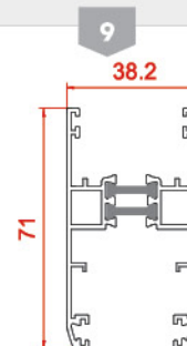
لنگه بدون زهوار Vent profiles 20850-20850 1.142 kg/m
