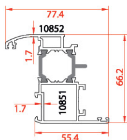
لنگه پنجره ضخامت ۱.۷ Vent profile 10851-10852 1.684kg/m
