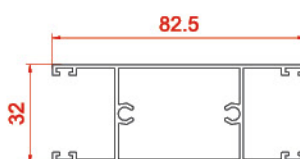
پروفیل سه پری بدون زهوار Tripetalous profiles
