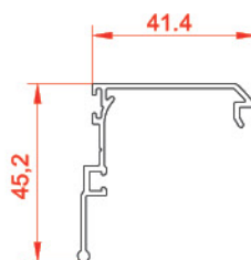
اینتر لاک inter lock for sliding vent 20067 weight: 0.436 kg/m
