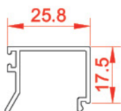
زهوار تک جداره 6 mm Glazing Bid 21657 0.261 Kg/m
