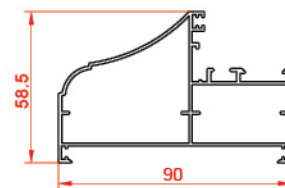
پروفیل کتیبه Cornice profiles
