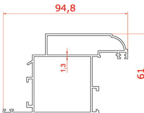
پروفیل لنگه داخل باز شو Inside Opening vent Profile 2606 1.3854 kg/m
