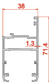
لنگه زهواردار Vent with rickity 21053 0.917 kg/m
