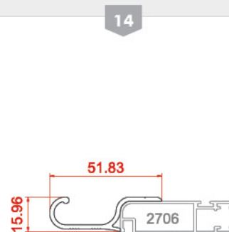
دستگیره لنگه توری Grid handle 21014 0.445 kg/m
