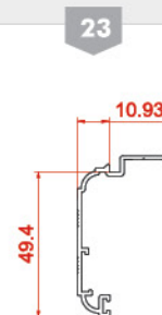
پروفیل روکوب Suppressed the blding 10319 0.422 kg/m
