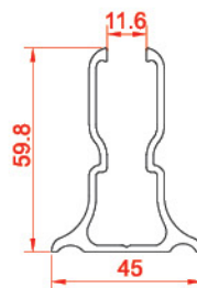
شیشه گیر Glass Holder 10468 1.111 kg/m
