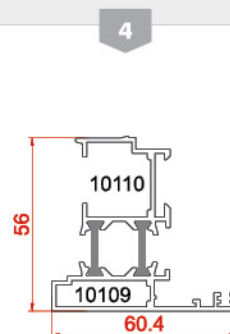
پروفیل وسط دولنگه The middle vent profiles 10109-10110 1.3 kg/m
