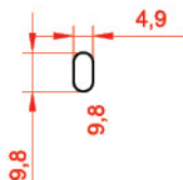
پروفیل زیر چرخ بلبرینگ Rail Profile
