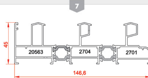
پروفیل فریم سه ریل 3 Rail frame 20563-2704-2701 2.59 kg/m
