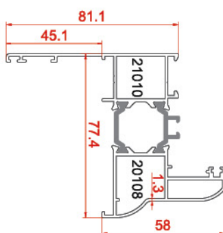
فریم روکوب دار Frame Profiles 21010-20108 1.739 kg/m
