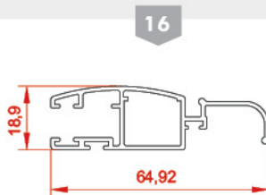
پروفیل کتیبه FRAME PROFILES 10196-10507 1.792 kg/m
