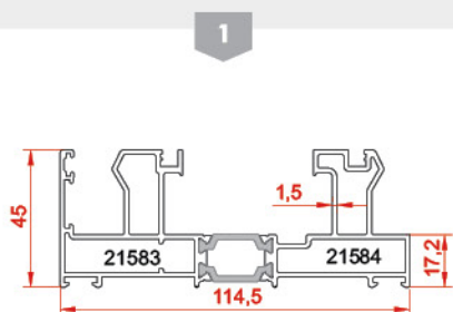
پروفیل فریم Frame Profile 21583-21584 weight: 2.254 kg/m
