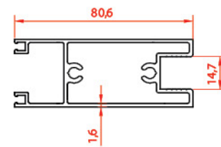
پروفیل ۸ سانتی 8cm profile 10810 1.372 kg/m
