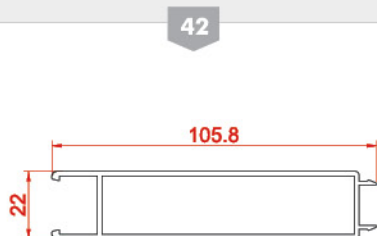
ورق دو جداره sheet Double 785 1.078 kg/m
