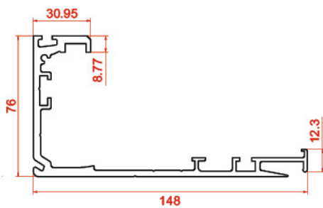
پروفیل ریل Rail profile 20780 3.146 kg/m
