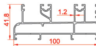
پروفیل فریم leftFrame Pro 21489 1.611 kg/m
