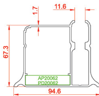
شیشه گیر Glass Holder 21496 2.217 kg/m
