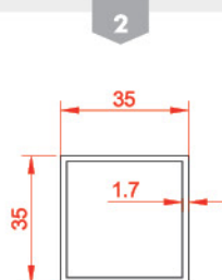
قوطی ۳۵ x ۳۵ Box 35x35 21653 0.649 Kg/m
