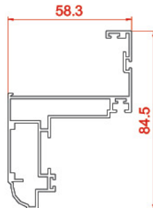
پروفیل دوجداره بازشو Double-glazed opening profiles 2749 1.1840 kg/m
