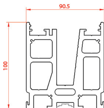
پروفیل شیشه گیر Glass stuck
