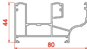
پروفیل فریم ریل دار rail grid with profiles Frame 2745 1.2444 kg/m
