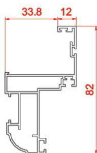
پروفیل دوجداره ثابت Fixed double Glazing profiles 2748 1.043 kg/m
