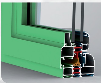
دیتیل یراق آلات پنجره لولایی ترمال بریک سری TH 75L Thermal break hinged window fittings of series TH 75L (detail)
