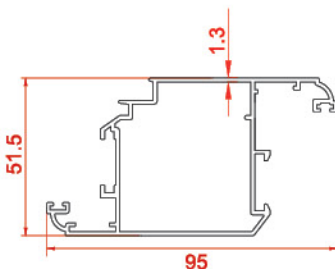
پروفیل لنگه Vent profiles 724 1.2656 kg/m
