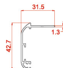
پروفیل روکوب ۴۲ Suppressed the bilding 10464 0.361 kg/m
