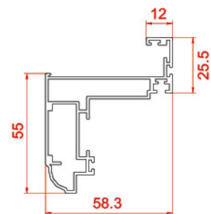
پروفیل یک جداره بازشو Single-walled opening profiles 10114 1.13 kg/m
