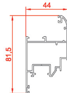
لنگه متوسط اسپانیولی Vent profile 21206 1.016 kg/m
