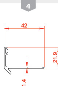
فریم نصب باز شو Opening Frame Profile 21655 0.315 Kg/m
