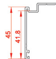
پروفیل روکوب Suppressed the blding 20564 0.328 kg/m
