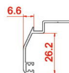
روکوب 3 سانتی Suppressed the binding 20031 0.2724 kg/m
