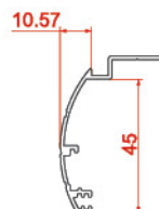
روکوب گرد Suppressed the binding 10117 0.380 kg/m
