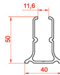
شیشه گیر Glass Holder 10490 0.863 kg/m
