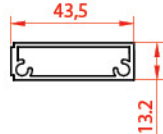
لقمه سپری T profile Pice 10514 0.515 kg/m
