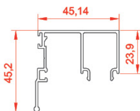
اینتر لاک در سپری فریم interlock for fix side 21624 weight: 0.626 kg/m
