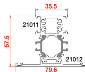
پروفیل سه پری تقویت شده Tripetalous profiles 21012-21011 2.193 kg/m
