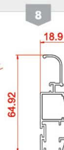
لنگه توری Grid vent 21076 0.634 kg/m
