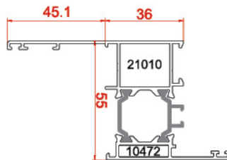
فریم روکوب دار Frame Profiles 10472-21010 1.421 kg/m
