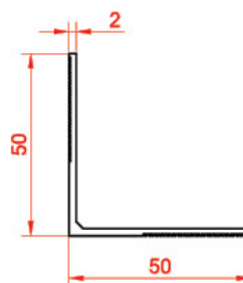
پروفیل 50X50 21217 0.531
