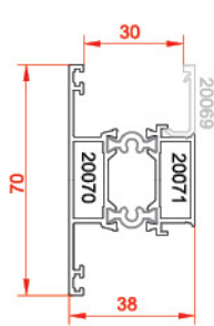
سپری برای ۲۱۲۲۳-۲۱۲۲۴ Tripetalous with rickety 20070-20071 0.936 kg/m
