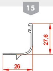
ریل توری Grid Rail 20777 weight: 0.230 kg/m
