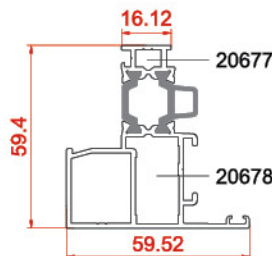
پروفیل لنگه Vent profiles 20677-20678 1.32 kg/m
