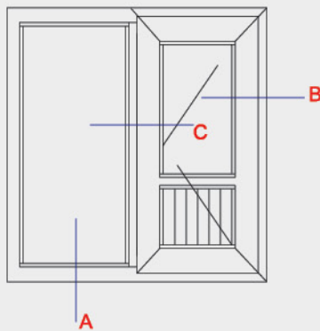
دیتیل یراق آلات درب آلدوکس سنگین AH45H طرح ایران Heavy Door aldoks fitting of series AH 45H Iran plans (detail)
