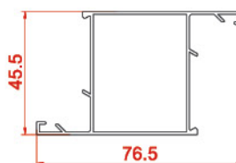
پروفیل لنگه Vent profiles 181 0.690 kg/m
