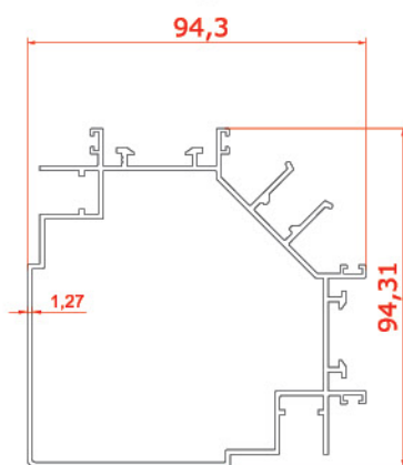
پروفیل پایه نود درجه دو طرفه By 90 Degrees Bilaterally 20928 1.859 kg/m
