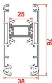
پروفیل لنگه زهوار Vent profiles 20659-20659 1.587 kg/m
