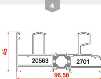
پروفیل فریم Frame profile 20563-2701 1.844 kg/m
