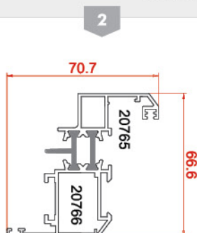
پروفیل لنگه جدید New Vent profiles 20765-20766 1.476 kg/m
