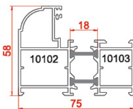
پروفیل فریم Frame profiles 10102-10103 1.783 kg/m
