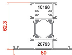
پروفیل سه پری لنگه Tripetalous Profiles 10198-20793 1.481 kg/m
