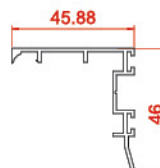
درپوش Gap 10136 0.4568 kg/m
