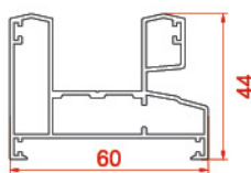
پروفیل فریم ساده profiles frame Simple 2744 1.049 kg/m
