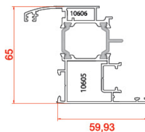
لنگه یراق یو پی وی سی پنجره Window vent 10605-10606 1.596 kg/m
