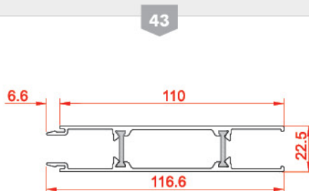
ورق دوجداره‌ی ترمال بریک Thermal break facade 21832-21832 1.409 kg/m
