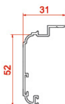
پروفیل روکوب ۵۲ Suppressed the bilding 10466 0.428 kg/m
