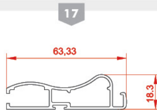
درپوش سه لنگه وسط باز شو cap for three sash sliding 21642 0.373 kg/m
