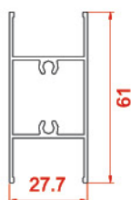
پروفیل سه پری Tripetalous profiles 754 0.7038 kg/m
