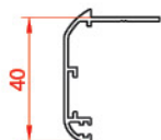
پروفیل روکوب Suppressed the binding 10464 0.352 kg/m
