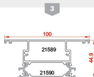
پروفیل سپری Sliding sash transom-mullion profile 21589-21590 weight: 1.636 kg/m
