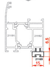
پروفیل نصب برس Plug insert for brushes
