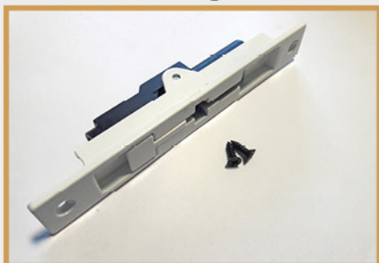
■ کد: 53076 قفل آکادئون سفید ■ کد: 53100 مشکی
